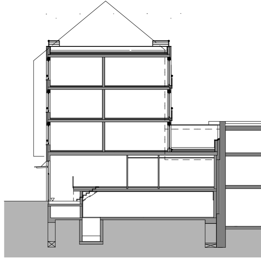
SCHNITT A-A
